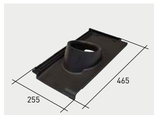
Q118*K | Teja soporte chimenea Innova/Vienna klinker
