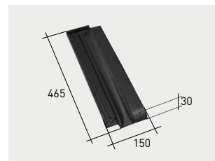
Q119*K | Media teja Innova klinker
