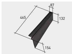
Q116*K | Remate lateral derecho Innova/Vienna klinker
