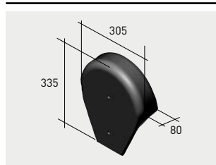
Q83*K | Tapón cumbreira circular klinker klinker
