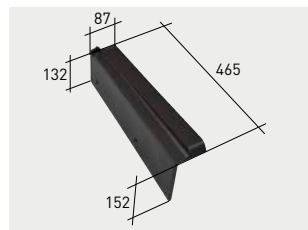
Q115*K | Remate lateral izquierdo Innova/Vienna klinker
