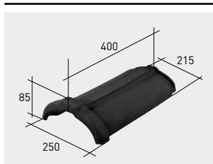
Q01*K | Cumbreira klinker
