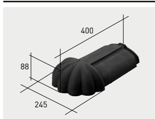
Q03*K | Remate cumbreira klinker
